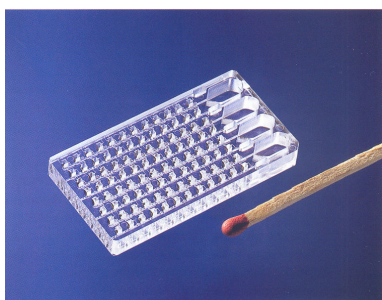
Obr. 7: Titrační mikrodoska - STEAG microParts GmbH, Německo (vlevo) a buňkové kontejnery s mechanicky vytvořenou vložkou – rozměr cca 300 x 300 x 300 \mu\text{m} , Forschungszentrum Karlsruhe, Německo (vpravo)
