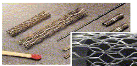
Obr. 12: Laserem vyrobený koronární stent s detailním pohledem (Forschungszentrum Karlsruhe, Německo)
