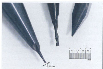
Obr. 6: Mikrofrézořovací nástroje od firmy Paul Horn GmbH (Německo)
